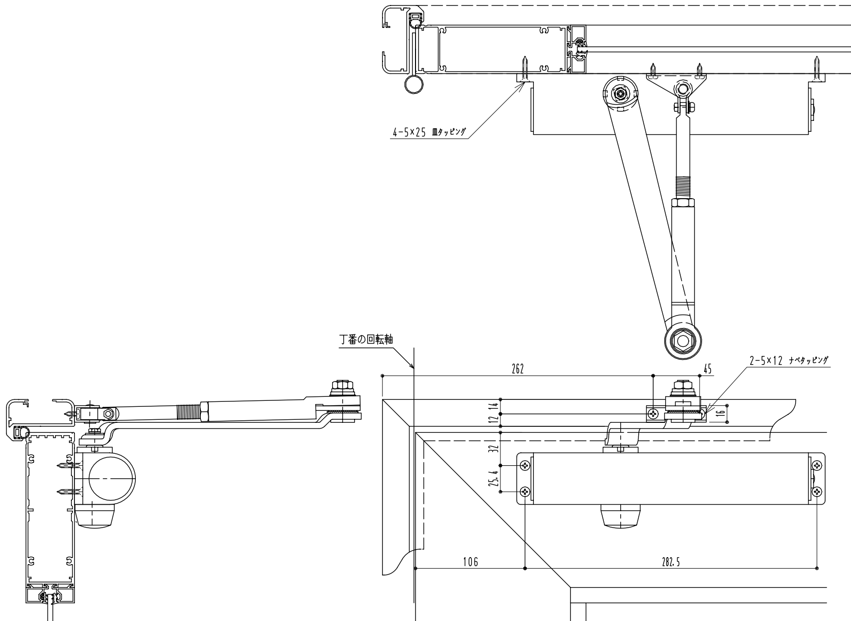
SUNWIZZ ドアクローザー 取付け寸法図 <DK40 - 左吊用 RYOBI表付け型 DS - 3000 >
