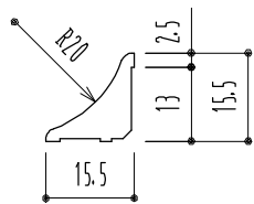
R巾木 20R-ABS L2000 (ABS樹脂 シルバー色)
