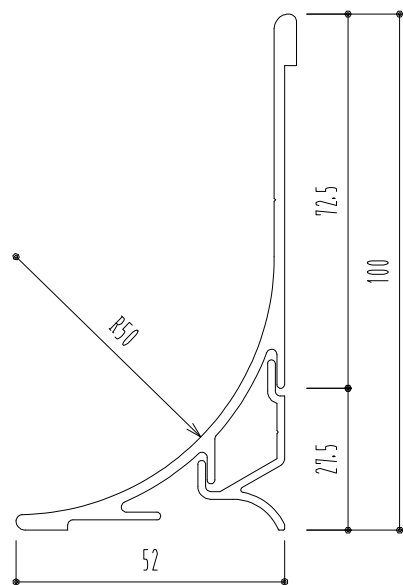
R巾木 50R-100SUS L3000 (ステンレス HL)
