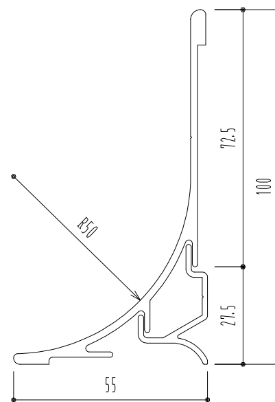
R巾木 50RF-100SUS L3000 (ステンレス HL)
