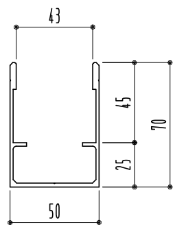
アルミ床レール 42-70HS L4000 (アルミ シルバー)
