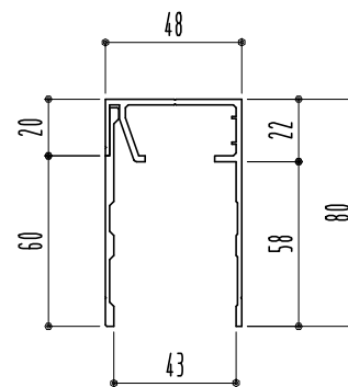
アルミ上部レール 42-TP80 L4000 (シルバー)
