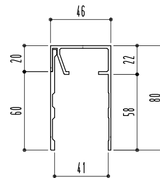
アルミ上部レール 40-TP80 L4000 (シルバー)
