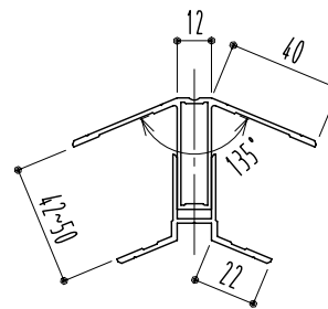
アルミ連結チャンネル CW135 L4000 (アルミ シルバー)
