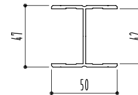
アルミ連結チャンネル CW180 L4300 (アルミ シルバー)
