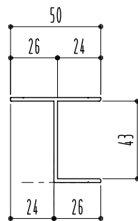
アルミ連結チャンネル TC42 L4000 (アルミ シルバー)
