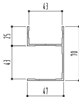
アルミ連結チャンネル CW90 L4000 (アルミ シルバー)
