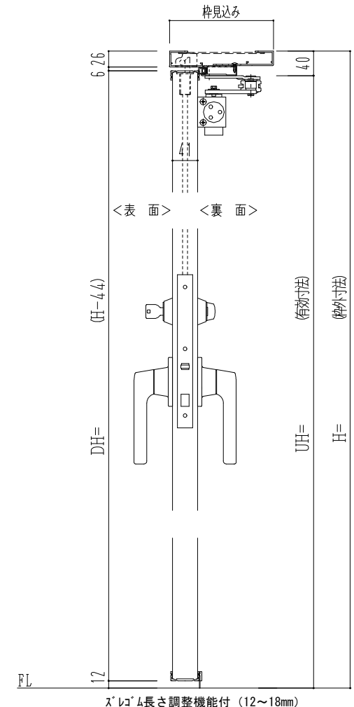
スレーム長さ調整機能付 (12~18mm)
