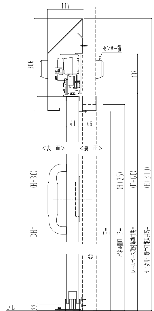
自動装置 ハング技研 EDM18NA
