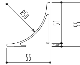
R中木 50R-55AL L3000 (アルミ シルバー)
