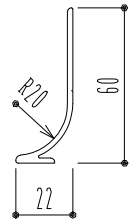
R中木 20R-60AL L3000 (アルミ シルバー)
