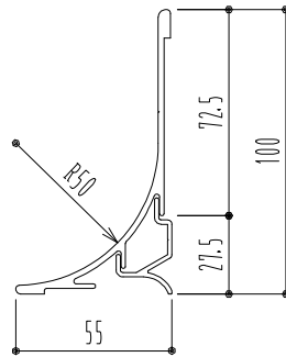
R中木 50RF-100AL L3000 (アルミ シルバー)
