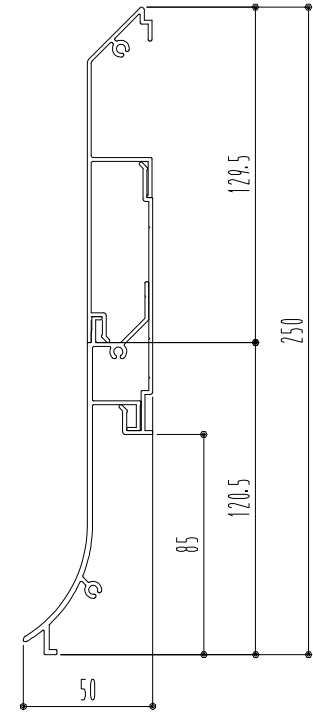
R中木 50R-250AL L3000 (アルミ シルバー)
