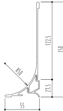
R中木 50RF-150AL L3000 (アルミ シルバー)
