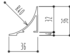
R中木 40R-AL L3000 (アルミ シルバー)
