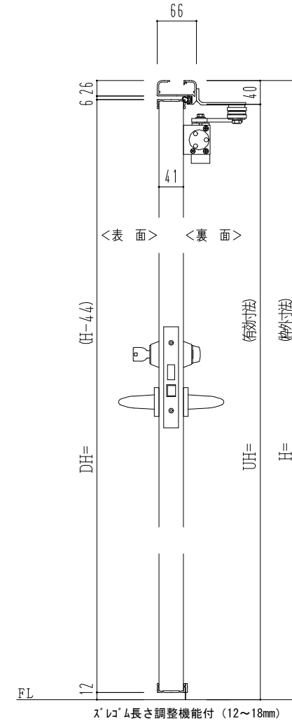
スレーム長さ調整機能付 (12~18mm)
