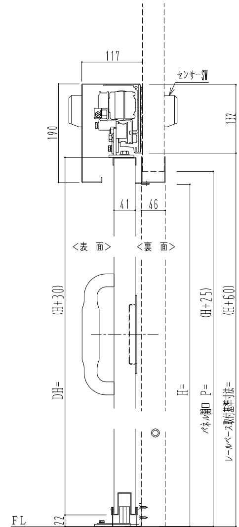
自動装置 ハング技研 EDM18NA
