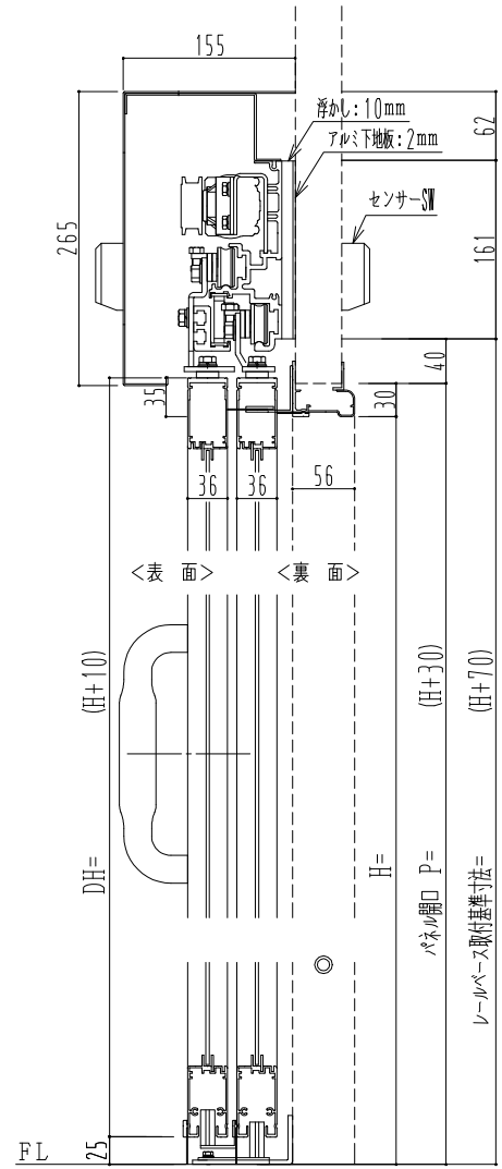
自動装置 ハンダ技研 EDM18A-2
